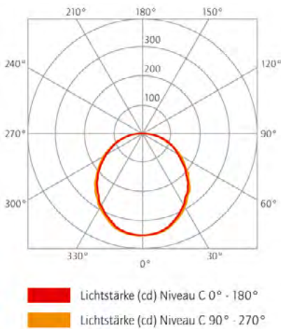
LICHTVERTEILUNGSKURVE 54 Watt (PL96La.5483.M.S1W0)
