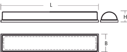
Bauform 011R
