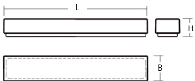
Bauform 011K.OD
