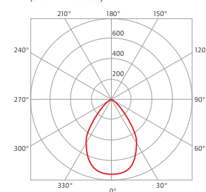
LICHTVERTEILUNGSKURVE 24 Watt (6152n.2440.A0.81)
