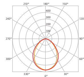
LICHTVERTEILUNGSKURVE 36 Watt (6030.3640.MPO.81)
