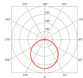
LICHTVERTEILUNGSKURVE 16 Watt (6014.1640.OP.81)
