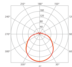
LICHTVERTEILUNGSKURVE 15 Watt (5280.1540.TO.80)
