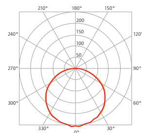
LICHTVERTEILUNGSKURVE 38 Watt (3842.3840.OP.80)
