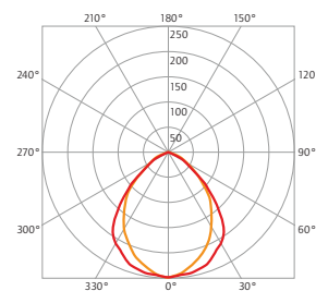
LICHTVERTEILUNGSKURVE 102 Watt (3790.10240.WO.81)
