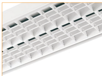
Raster durch Stahlstreben verstärkt und mit dem Leuchtkörper verschraubt
