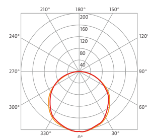
LICHTVERTEILUNGSKURVE 36 Watt (2840q.3640.OP.80)
