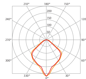
LICHTVERTEILUNGSKURVE 20 Watt (2820.2040.AW.80)
