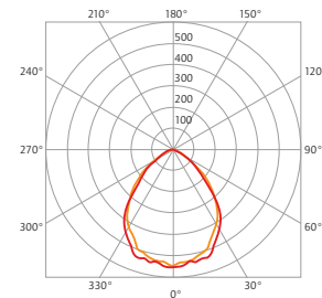
LICHTVERTEILUNGSKURVE 40 Watt (2720.4040.DO.80)
