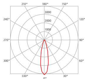
LICHTVERTEILUNGSKURVE 3 Watt (2684L.340.LO.80)
