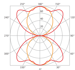
LICHTVERTEILUNGSKURVE 52 Watt (2530i.5240.MP.80)
