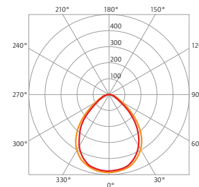
LICHTVERTEILUNGSKURVE DIREKT 43 Watt (2170.4340.MPI.80)
