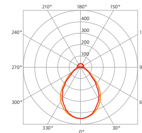
LICHTVERTEILUNGSKURVE DIREKT/INDIREKT 43 Watt (2170.4340.MPI.80)
