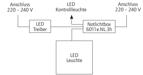
Notlichtkit 6011e.NL.3h
