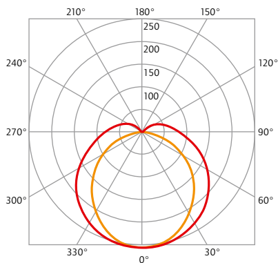
LICHTVERTEILUNGSKURVE 24 Watt (7114.2440.PC.80/IN)
